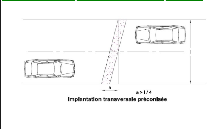
2.2.2 - Schéma d'implantation transversale préconisée
