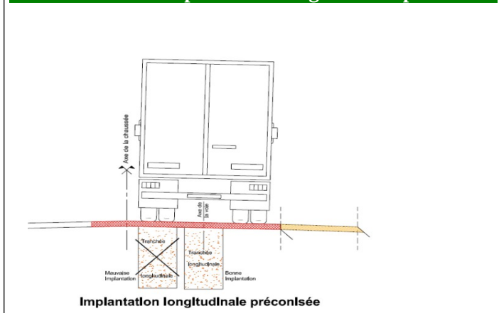
2.2.1 - Schéma d'implantation longitudinale préconisée
